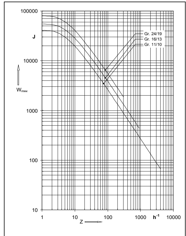
Abb. 33/1: Höchst-Schaltarbeit W_{\max} pro Schaltung in Abhängigkeit von der stündlichen Schaltzahl Z ; (Werte gelten für n=1500 \text{ min}^{-1} )
